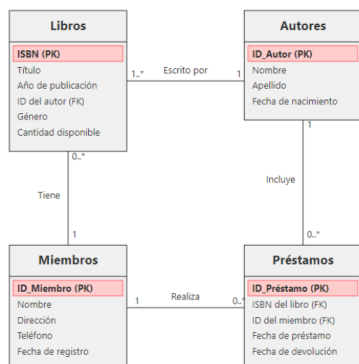
Diseño - Entidad-relación
