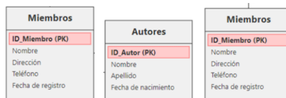
Diseño - Lógico
